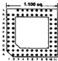
Footprint 11034
