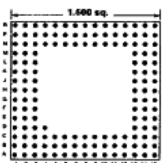
145 PINS Footprint 15024
