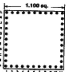
Footprint 11044
