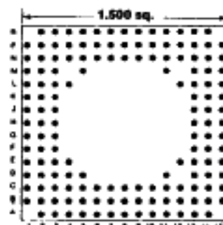
149 PINS Footprint 15019
