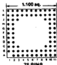
Footprint 11016
