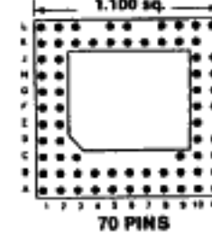
Footprint 11028
