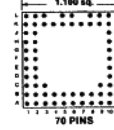
Footprint 11029
