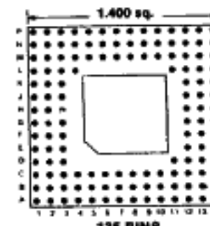
135 PINS Footprint 14011
