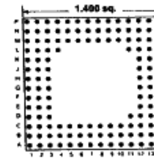
135 PINS Footprint 14012
