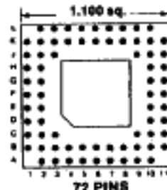
Footprint 11026
